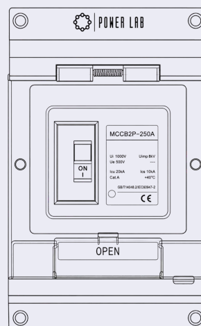
MCCB 125A-250A
