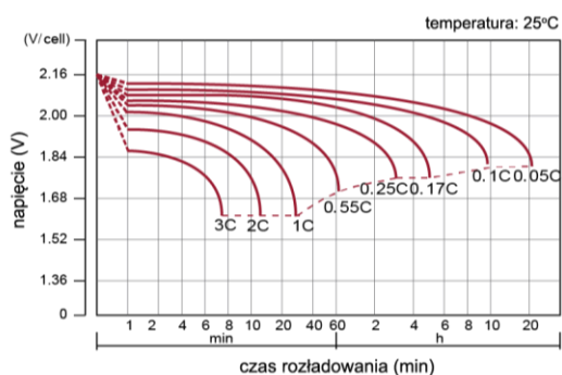
CHARAKTERYSTYKA ROZŁADOWANIA
